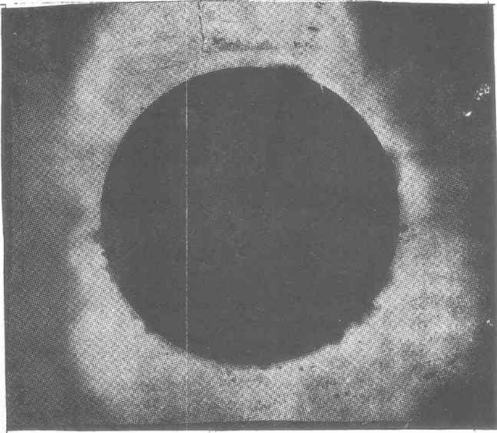
سورج گرہن کا ایک منظر - ماؤنٹ وین رصد گاہ - ۱۸ جون ۱۹۱۸ء
