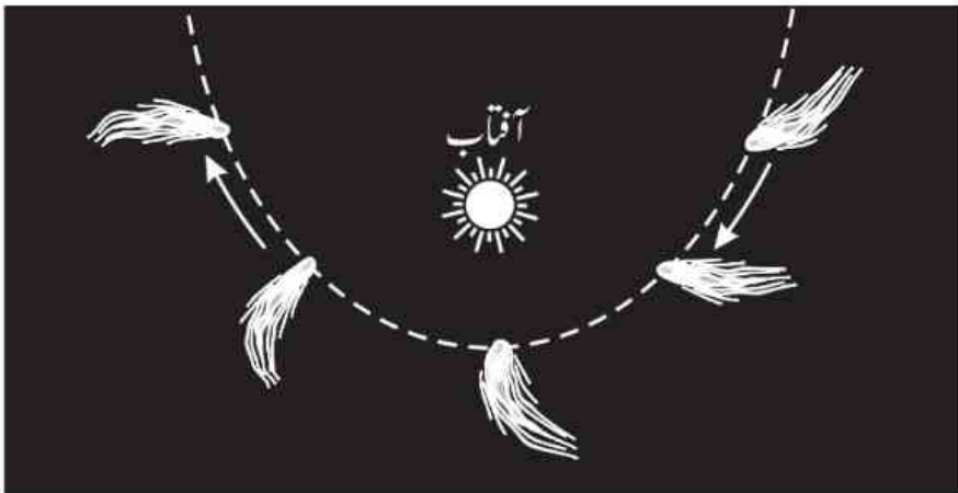
دُمدار کی دم کے مظاہر
