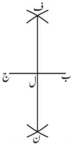
شکل عمود و تنصیف خط مستقیم
