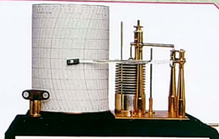
مَرَسَمَةُ الضَّغْطِ بارو گراف Barograph
